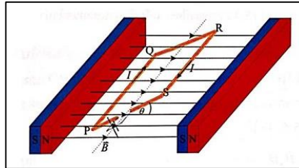
รูป 15.40 ระนาบขดลวดทำมุม \theta กับสนามแม่เหล็ก
