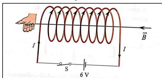
รูป 15.19 การหาทิศทางสนามแม่เหล็กของโซเลนอยด์โดยใช่มือขวา
