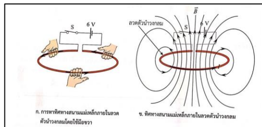
รูป 15.14 สนามแม่เหล็กรอบลวดตัวนำวงกลมเมื่อระนาบขดลวด อยู่ในแนวขนานกับระนาบระดับและมีกระแสไฟฟ้าผ่าน
