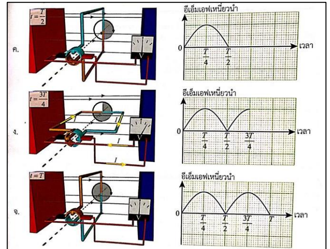
รูป 15.51 การหมุนของเครื่องกำเนิดไฟฟ้ากระแสตรง จาก 0 ถึง T และอีเอ็มเอฟเหนี่ยวนำที่เกิดขึ้น
