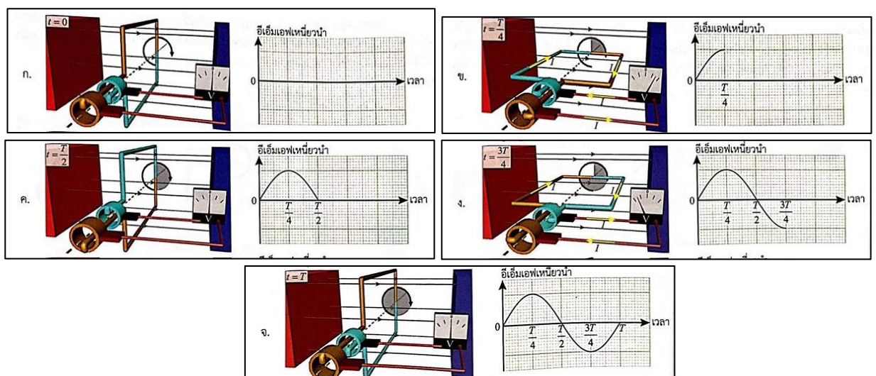
รูป 15.49 การหมุนของเครื่องกำเนิดไฟฟ้ากระแสสลับ 0 ถึง T และกราฟอีเอ็มเอฟที่เกิดขึ้น
