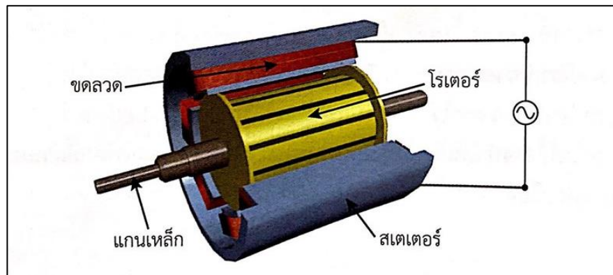
รูปแสดงส่วนประกอบของมอเตอร์ไฟฟ้าเหนี่ยวนำ
