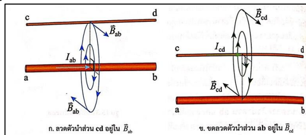
รูป 15.33 สนามแม่เหล็กที่เกิดจากกระแสไฟฟ้า I_{ab} ผ่านขดลวดตัวนำส่วน ab และสนามแม่เหล็กที่เกิดจากกระแสไฟฟ้า I_{cd} ผ่านลวดตัวนำส่วน cd
