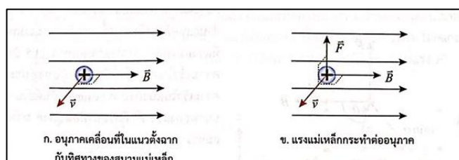
รูป 15.27 แรงแม่เหล็กที่กระทำต่ออนุภาคที่มีประจุไฟฟ้าและเคลื่อนที่ตั้งฉากกับสนามแม่เหล็ก
