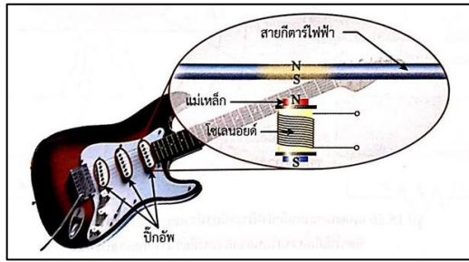
รูป 15.55 แสดงขั้วคอยล์ที่ใช้กับกีตาร์เพื่อรับสัญญาณไฟฟ้าจากการสั่นของสายกีตาร์
