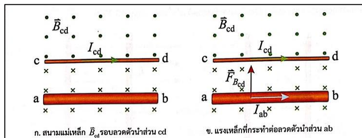
รูป 15.35 แรงแม่เหล็กจากสนามแม่เหล็กของลวดตัวนำส่วน cd ที่กระทำต่อขดลวดตัวนำส่วน ab
