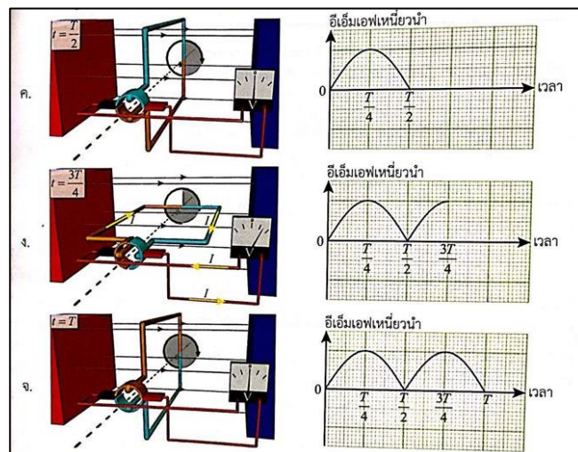
รูป 15.51 การหมุนของเครื่องกำเนิดไฟฟ้ากระแสตรง จาก 0 ถึง T และอีเอ็มเอฟเหนี่ยวนำที่เกิดขึ้น
