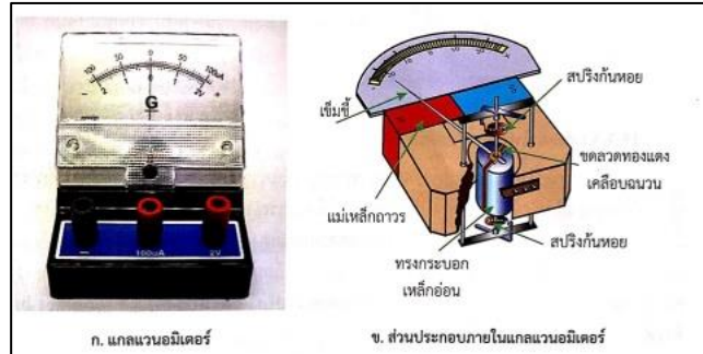
รูป 15.42 แกลแวนอมมิเตอร์และส่วนประกอบภายในแกลแวนอมมิเตอร์
