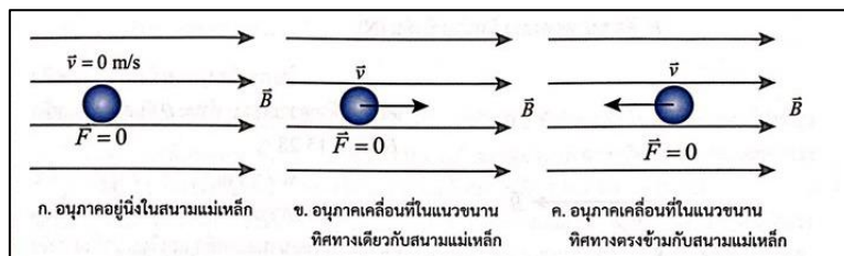
รูป 15.26 แรงแม่เหล็กที่กระทำต่ออนุภาคที่มีประจุไฟฟ้าที่อยู่นิ่งหรือเคลื่อนที่ขนานกับสนามแม่เหล็กมีค่าเป็นศูนย์
