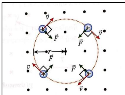
รูป 15.29 อนุภาคที่มีประจุไฟฟ้าบวกเคลื่อนที่แบบวงกลมในสนามแม่เหล็ก
