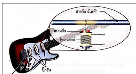
รูป 15.55 แสดงปิ๊กอัพที่ใช้กับกีตาร์เพื่อรับสัญญาณไฟฟ้าจากการสั่นของสายกีตาร์
