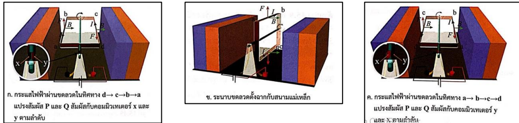
รูป 15.44 แรงกระทำต่อขดลวดของมอเตอร์ไฟฟ้ากระแสตรง
