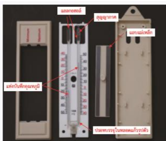
รูปส่วนประกอบของเทอร์มอมิเตอร์แบบขีดสเกลสำหรับวัดอุณหภูมิสูงสุดและต่ำสุด
