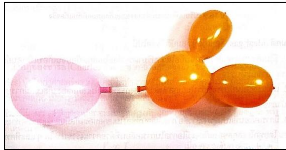
รูป 16.8 แก๊สเปลี่ยนปริมาตรตามรูปร่างของลูกโป่ง
