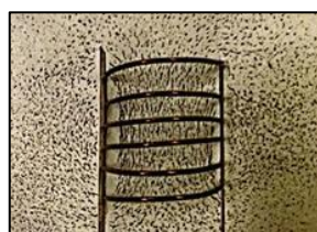
รูป 15.16 การเรียงตัวของผงเหล็กเมื่อมีกระแสไฟฟ้าผ่านโซเลนอยด์
