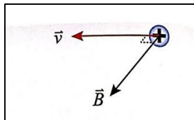
ก.อนุภาคที่มีประจุไฟฟ้าบวกเคลื่อนที่ในทิศทางตั้งฉากกับสนามแม่เหล็ก
