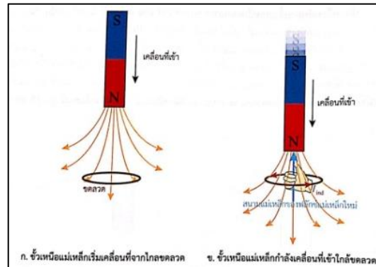
รูป 15.47 การเกิดอีเอ็มเอฟเหนี่ยวนำและกระแสเหนี่ยวนำในขดลวดเมื่อฟลักซ์แม่เหล็กเพิ่มขึ้น
