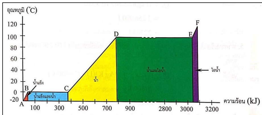
รูป 16.6 การเปลี่ยนถนของน้ำมวล 1 กิโลกรัม เมื่อได้รับความร้อน
