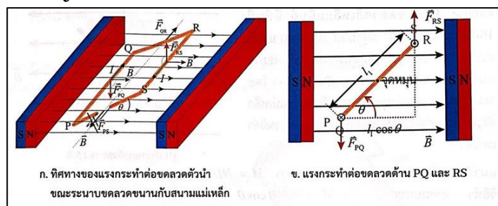
รูป 15.41 ขดลวดตัวนำสี่เหลี่ยมฉากเอียงทำมุมกับสนามแม่เหล็กและมีกระแสไฟฟ้าผ่าน
