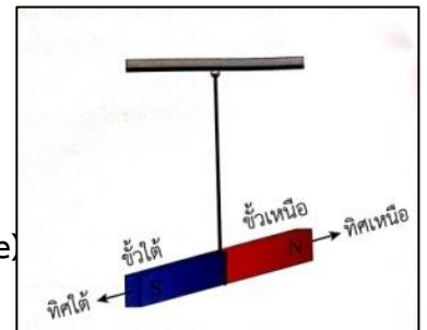
รูป 15.1 แท่งแม่เหล็กจะวางตัว ในแนวทิศเหนือ-ทิศใต้เสมอ
