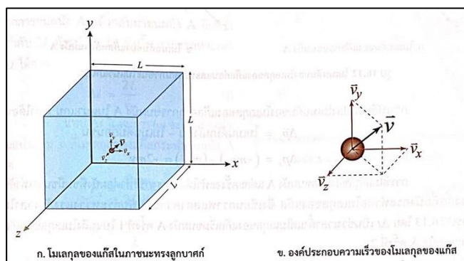
รูป 16.11 การเคลื่อนที่ของโมเลกุลของแก๊สในภาชนะทรงลูกบาศก์
