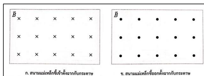
รูป 15.20 การใช้สัญลักษณ์ \times และ \cdot แสดงทิศทางของสนามแม่เหล็ก
