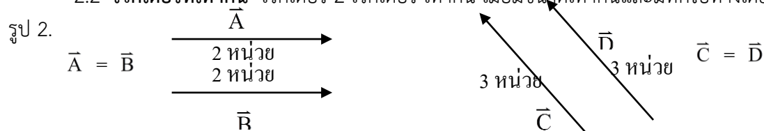
รูป 2. แสดงเวกเตอร์ที่เท่ากัน
