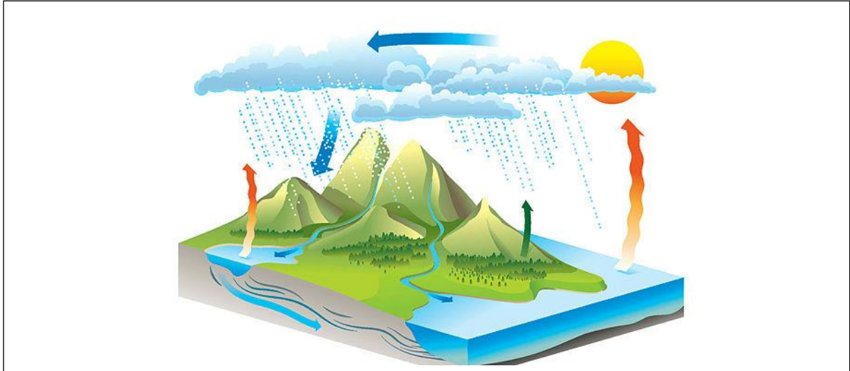
แผนภาพแสดงวัฏจักรทางอุทกวิทยา
